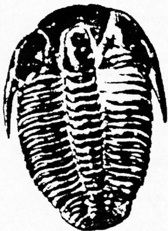
Trilobite
