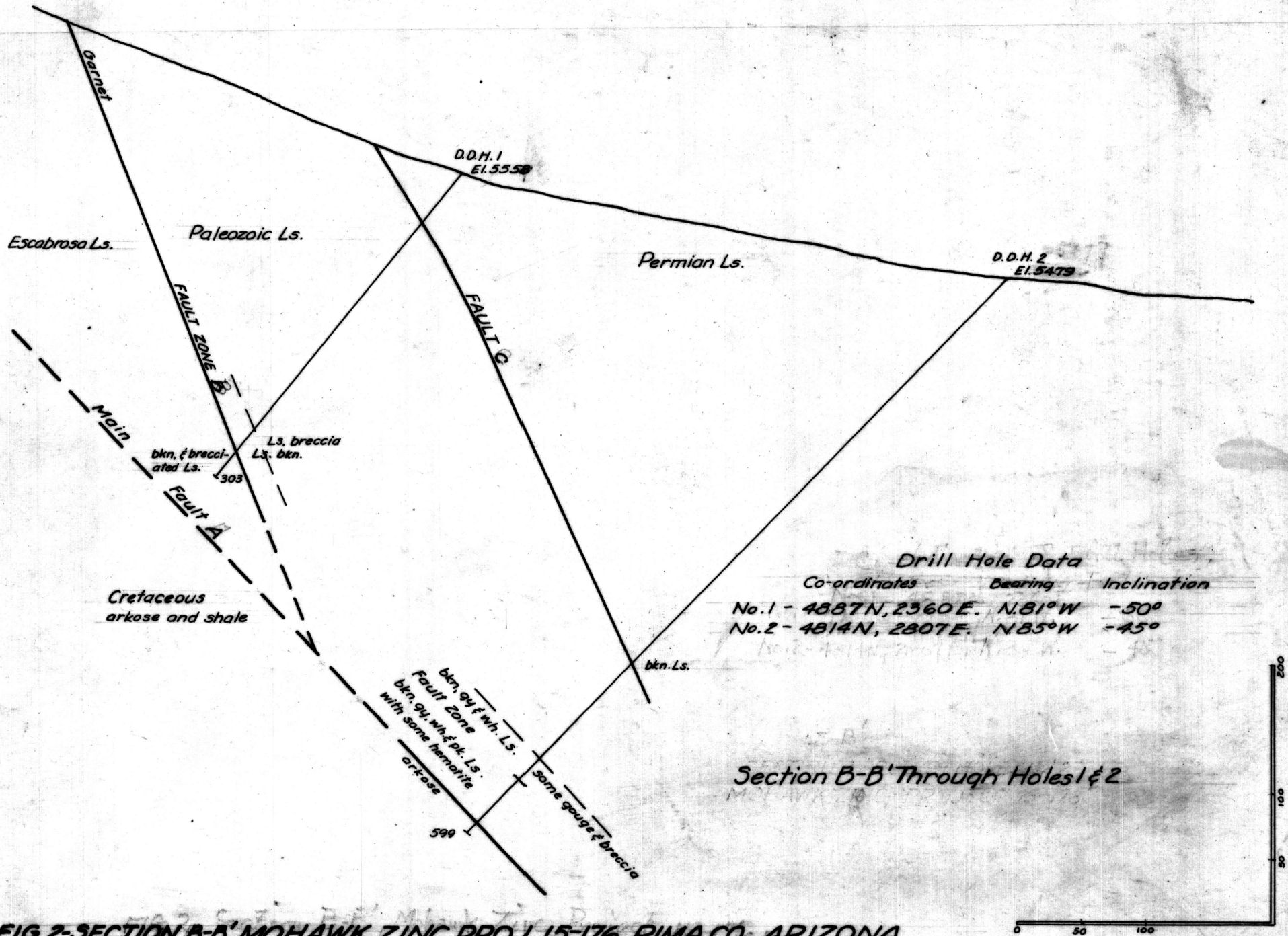
FIG. 2-SECTION B-B', MOHAWK ZINC, PROJ. 15-176, PIMA CO., ARIZONA
