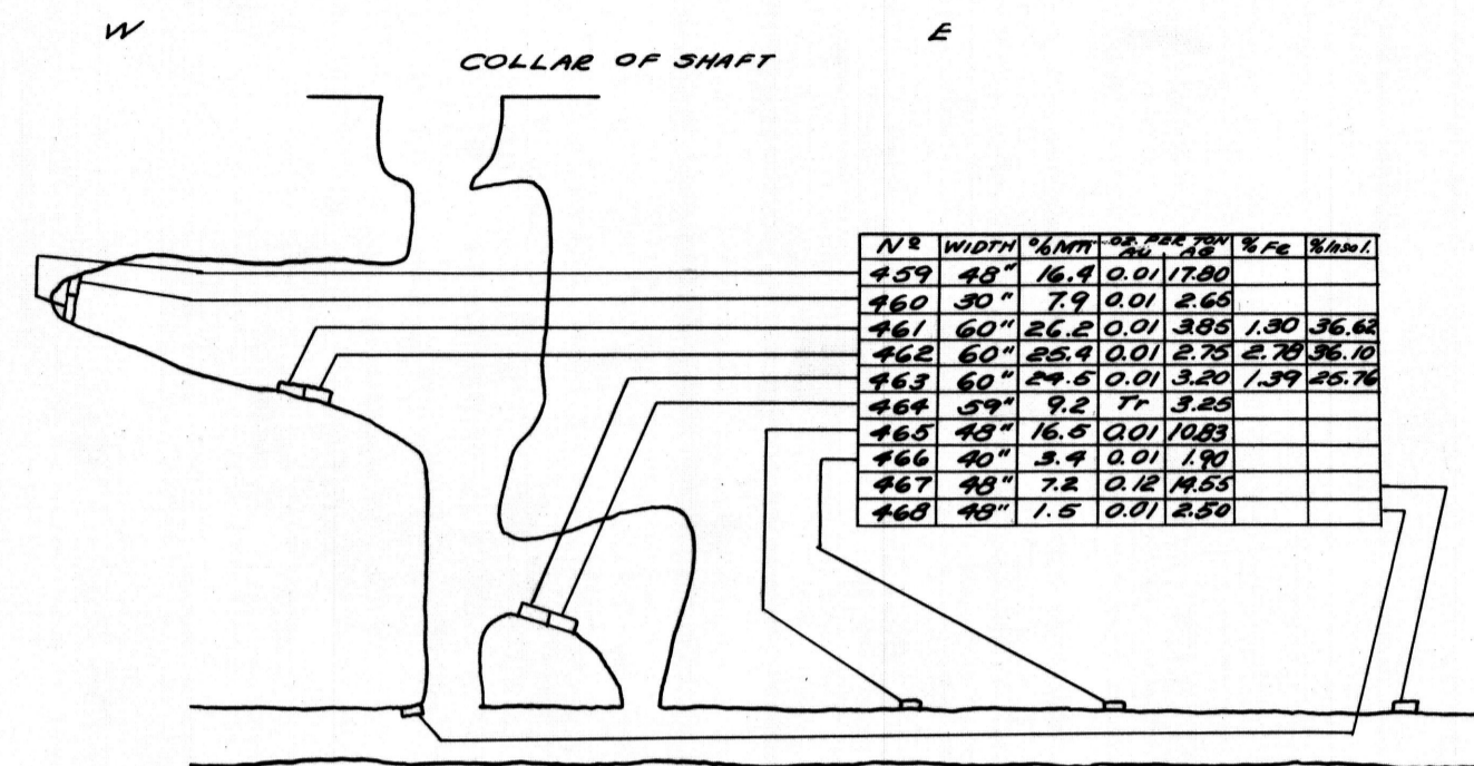
SECTION A-A' RATTLESNAKE SHAFT SCALE: 1"=40'
