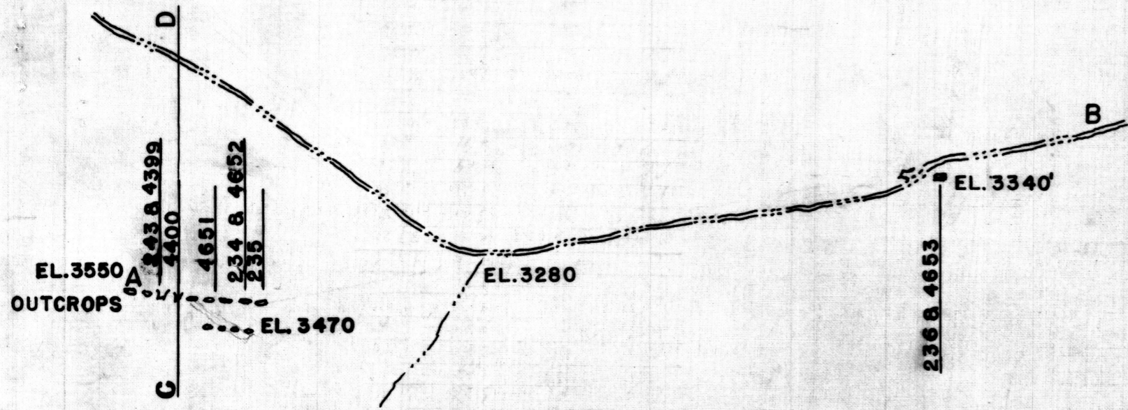
FIG. 1, PLAN
