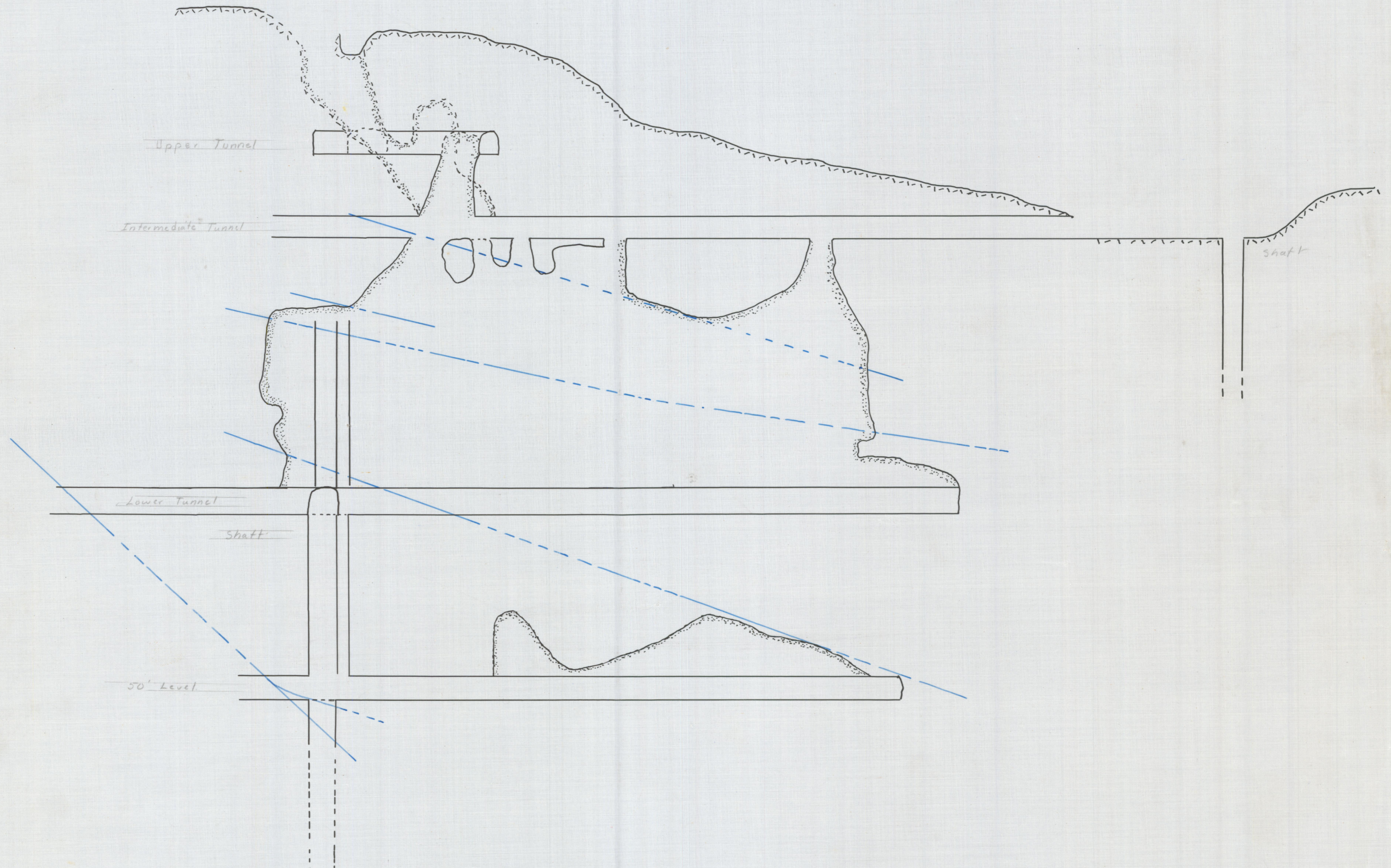
LONGITUDINAL SECTION
